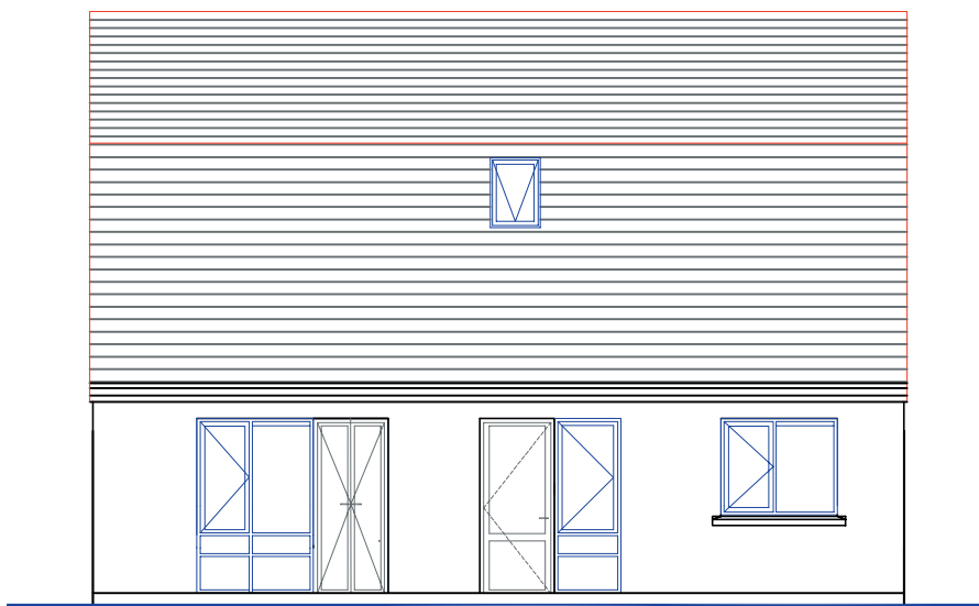
RERE ELEVATION
